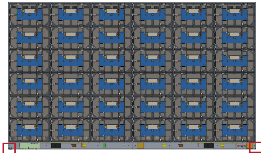
Системная плата управления
